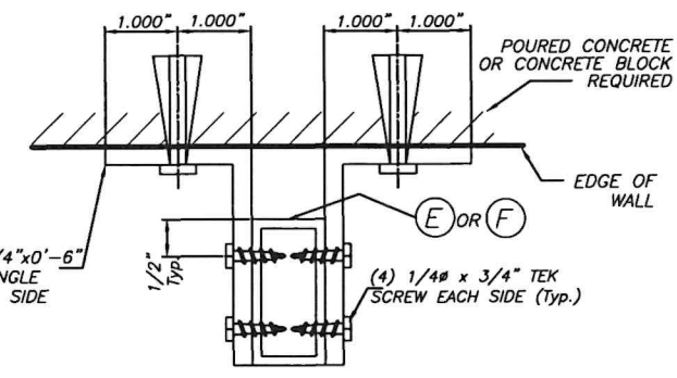
SECTION S1 - S1 SCALE : N. T. S.
